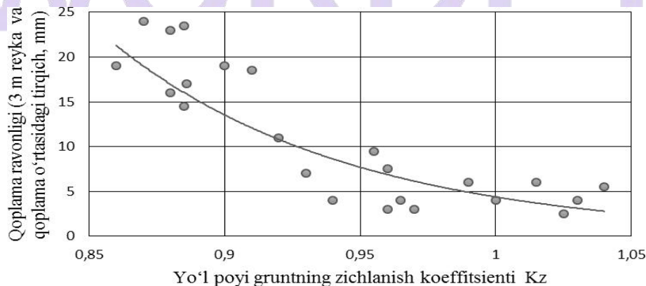
1.3-rasm. Qoplama ravonligi va yo'l poyi gruntining zichlanish darajasining o'zaro bo'g'liqlik grafigi.(Muallif tomonidan ishlab chiqilgan)
